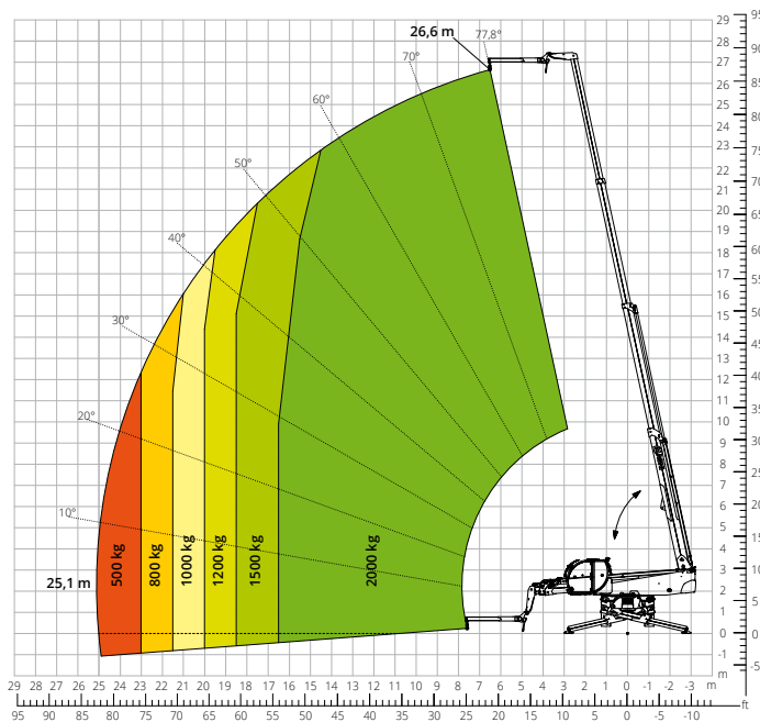
Abaque de charge avec PANIER NACELLE EXTENSIBLE ROTATIF 1 000 kg ATT - 01 - 016
