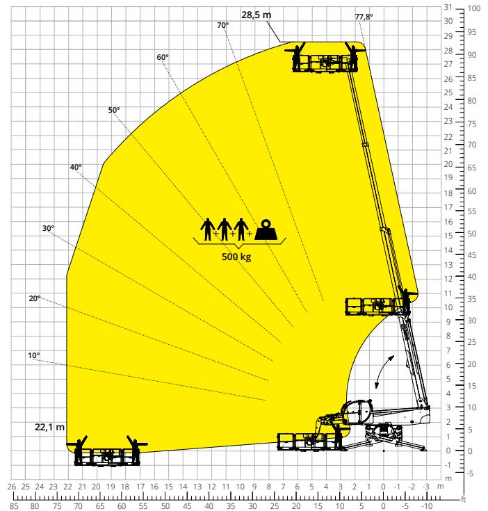
Abaque de charge avec PANIER NACELLE 500 kg AVEC TREUIL 600 kg ATT - 01 - 026
